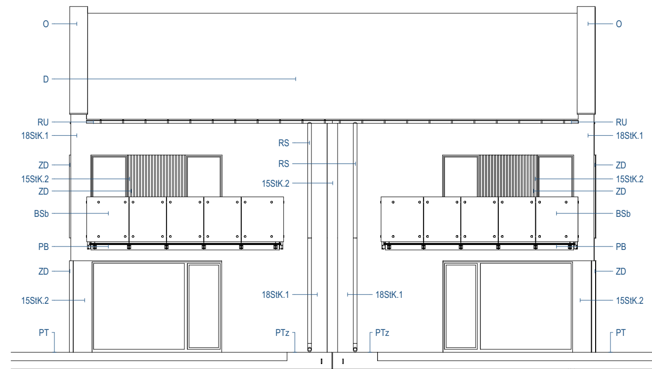
E-Wsch Elewacja Wschodnia 1:100
