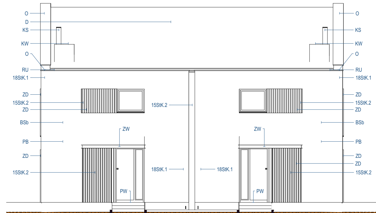
E-Zach Elewacja Zachodnia 1:100
