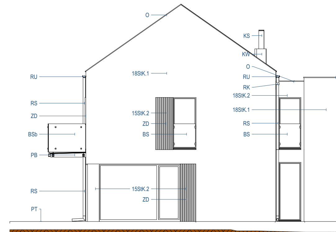
E-Pn Elewacja Północna 1:100
