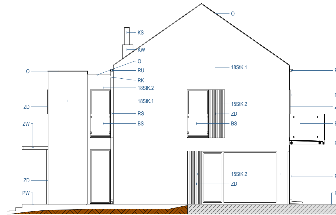
E-Pd Elewacja Południowa 1:100
